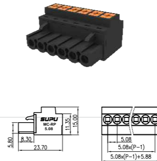
MC-RP5.08HXXP
