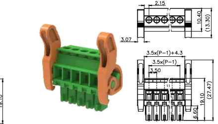
MC-RE3.5VXXC-I-0001
