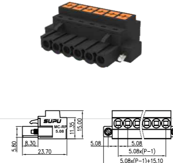
MC-RP5.08HXXP-I
